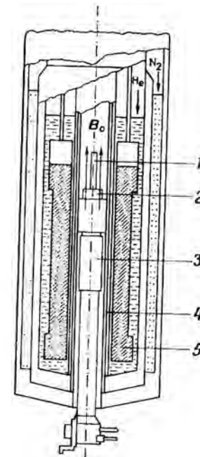
Рис. IX. 1. Схематическое изображение магнита со сверхпроводящим соленоидом [1].
