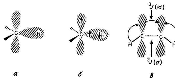
Рис. IV. 27. Схематическое представление \pi -механизма спин-спиновой взаимодействия между протонами.
