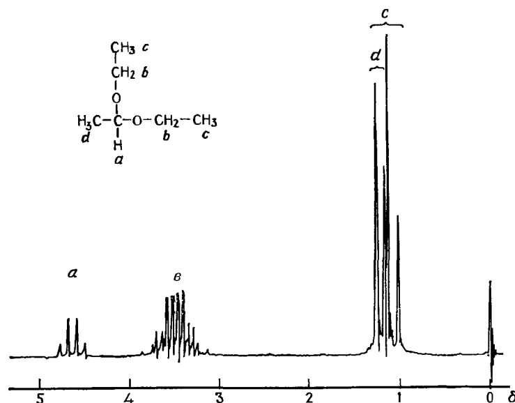
Рис. VI. 7. Спектр ЯМР (60 МГц) диэтилацетальа ацетальдегида.
