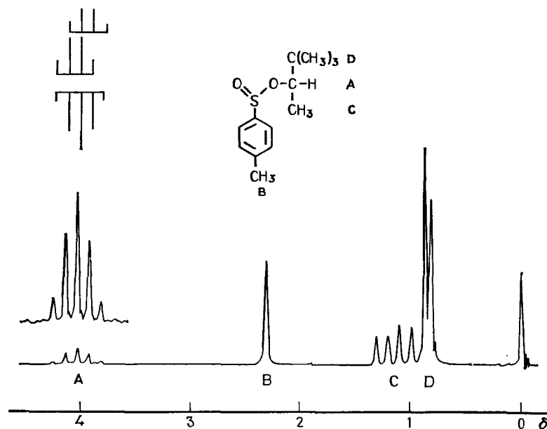
Рис. VI.5. Спектр ЯМР (60 МГц) продукта взаимодействия рацемического p -толуолсульфонилхлорида с ( S )-3,3-диметилбутанолом-2 (Рабан и Мнслоу [3]).
