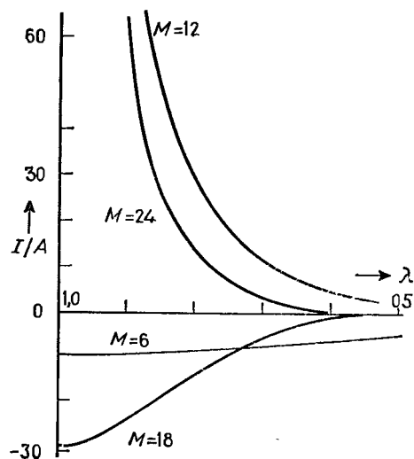
Рис. IV.15. Интенсивность кольцевого тока I на единицу площади A в аниуленах в зависимости от параметра альтернирования \lambda . (Попл, Уич [4].) \lambda является мерой отношения резонансных интегралов \beta для соседних углерод-углеродных связей. Для полностью эквивалентных связей \lambda = 1 . Отрицательный знак соответствует диамагнетизму. M — число присутствующих \pi -электронов.
