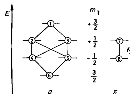
Рис. V. 7. Диаграмма энергетических уровней системы AB_2 . а — симметричное состояние; б — антисимметричное состояние.
