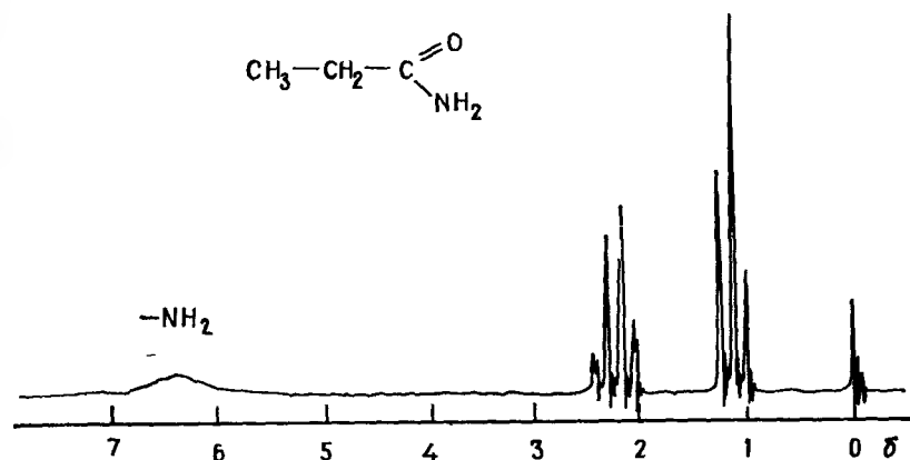
Рис. II. 8. Спектр протонного магнитного резонанса пропионамида.
