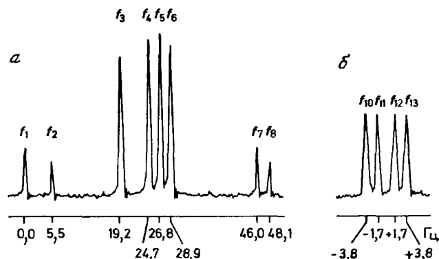
Рис. V.11. ABX-спектр протонов 4-бром-3-трет-бутилциклопентен-2-она (91); 60 МГц [2].
