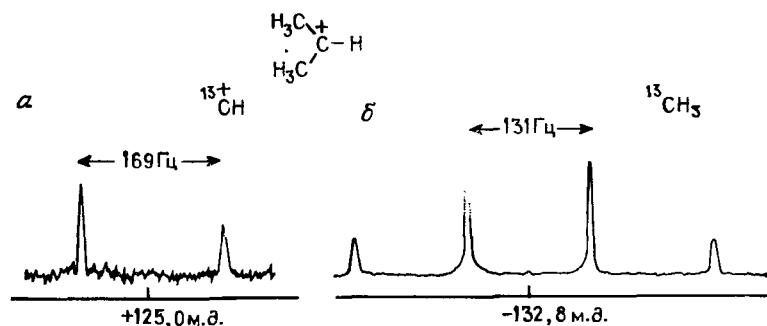
Рис. IX. 18. ^{13}\text{C} -ИНДОР-спектр изопропил-катиона.
