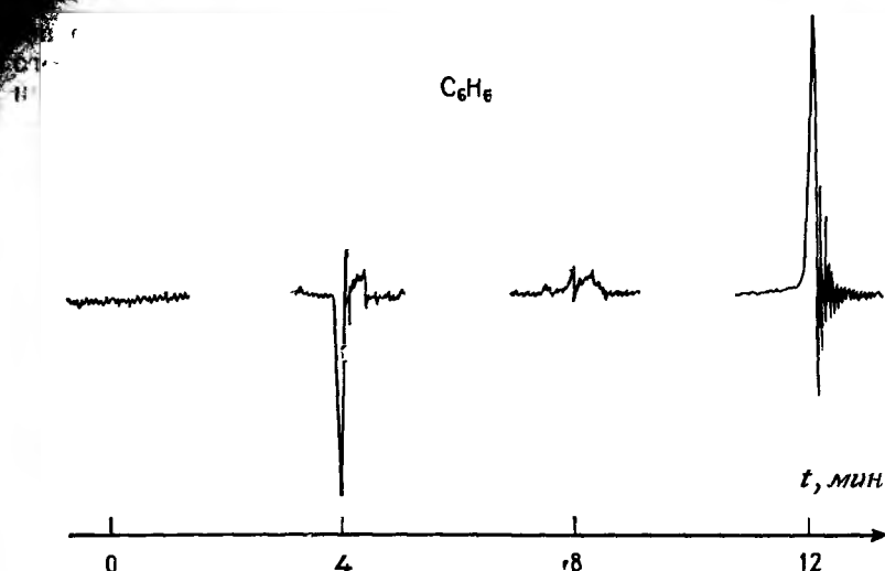
Рис. 4. Изменение вида спектра протонов бензола при термическом распаде бензоилпероксида в зависимости от времени проведения реакции.
