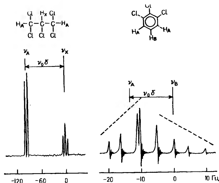
Рис. II. 20. Спектры протонного магнитного резонанса 1,1,2,3,3-пентахлорпропана и 1,2,3-трихлорбензола.
