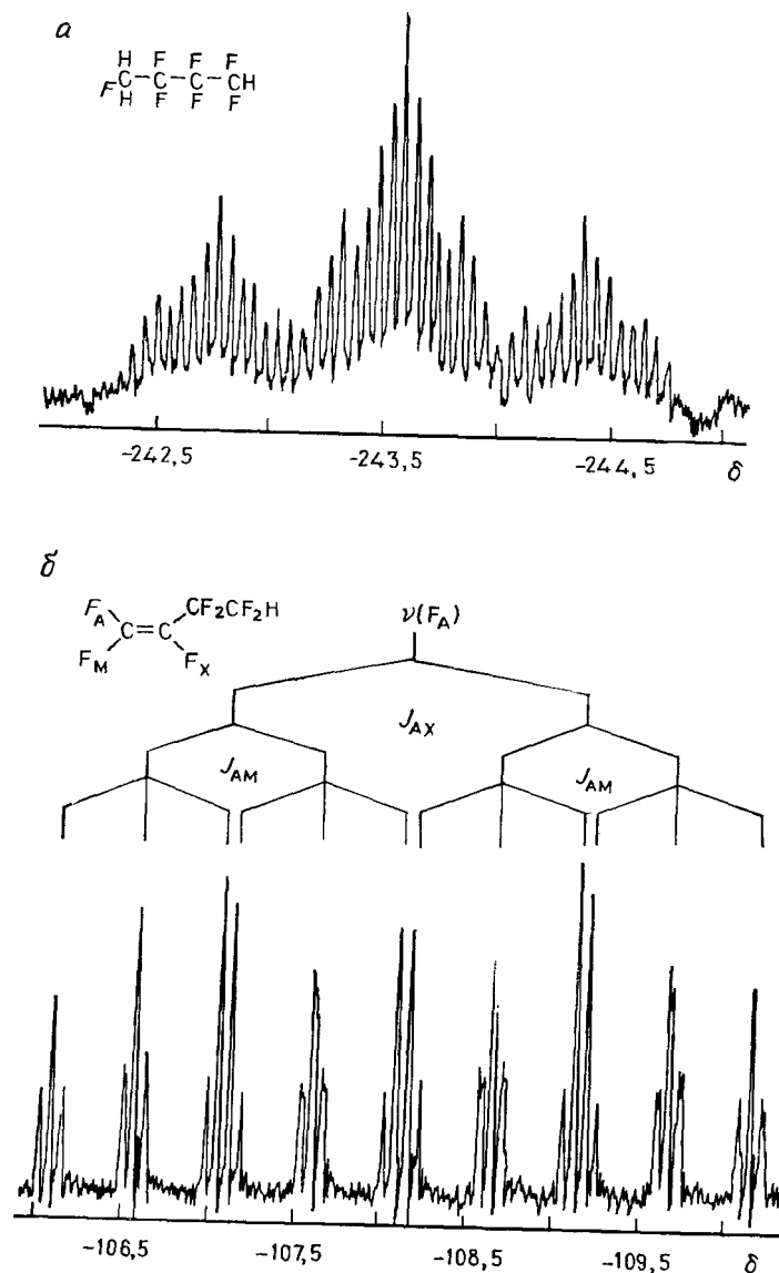
Рис. X. 4. Фрагменты спектров ЯМР ^{19}\text{F} 1H,1H,4H-гептафторбутана и 4H-гептафторбутена-1 (Муни [1]).
