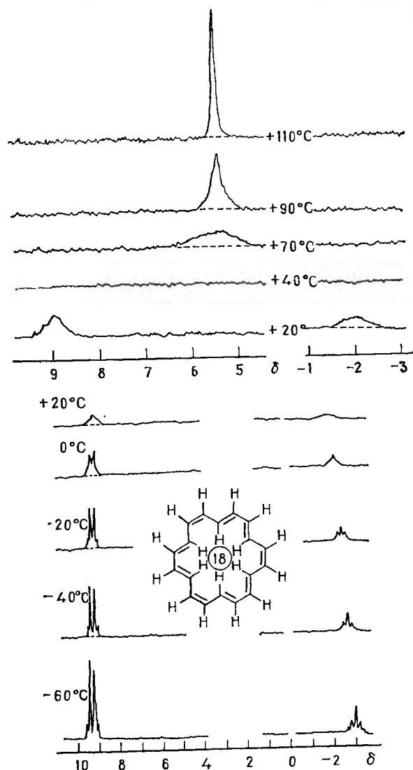
Рис. VIII.11. Температурная зависимость спектра ЯМР [18]аннулена (Хеймер и сотр. [6]).
