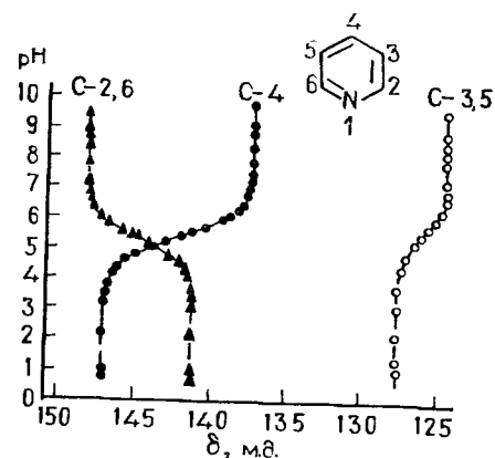
Рис. X. 18. Зависимость положения сигналов в спектре пиридина от pH раствора (Брайтмаер, Спон [13]).
