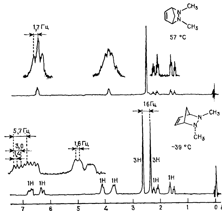
Рис. VIII.7. Температурная зависимость спектра ЯМР ^1\text{H} 2,3-дизабицикло[2.2.1]гептена-5 (147) (Андерсон, Лей [2]).
