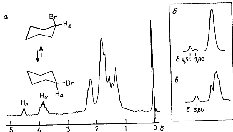
Рис. VIII.10. Спектры ЯМР монозамещенных циклогексанов. a — равновесная смесь аксиального и экваториального бромциклогексанов при -100^\circ\text{C} [4]; b — смесь аксиального и экваториального хлорциклогексанов при -150^\circ\text{C} (Дженсен, Башвиллер [5]); a — чистый экваториальный хлорциклогексан при -150^\circ\text{C} [5].
