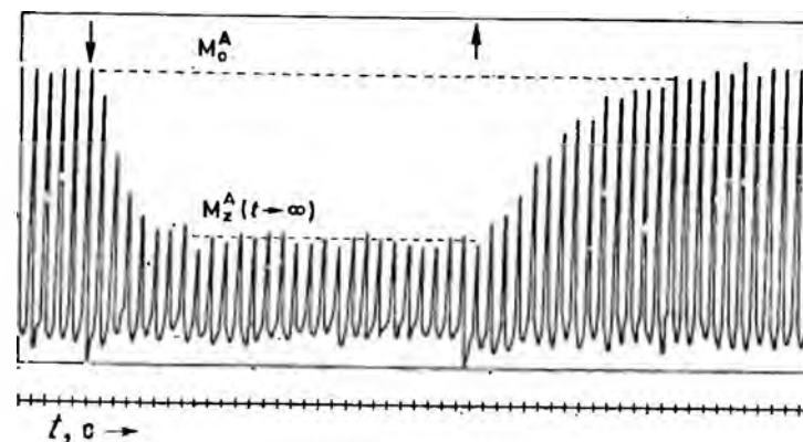
Рис. IX. 11. Изменение интенсивности сигнала гидроксильного протона 2-гидроксиацетофенона (189) как функция времени после включения и выключения поля B_2 с частотой OH-резонанса салицилового альдегида (190) (Форзен, Гоффман [7]).
