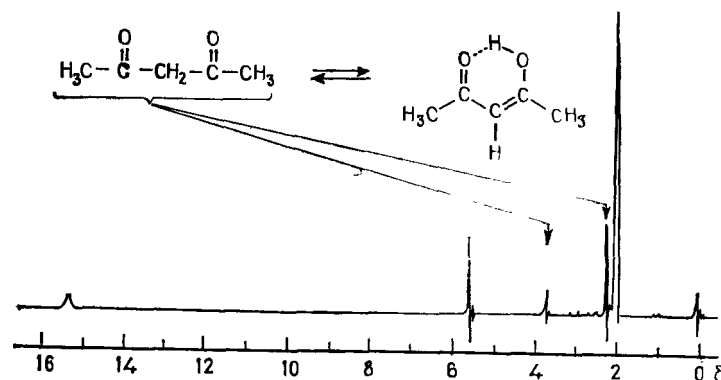
Рис. VIII.19. Спектр ЯМР 1 H ацетилацетона в растворе CCl 4 при комнатной температуре.
