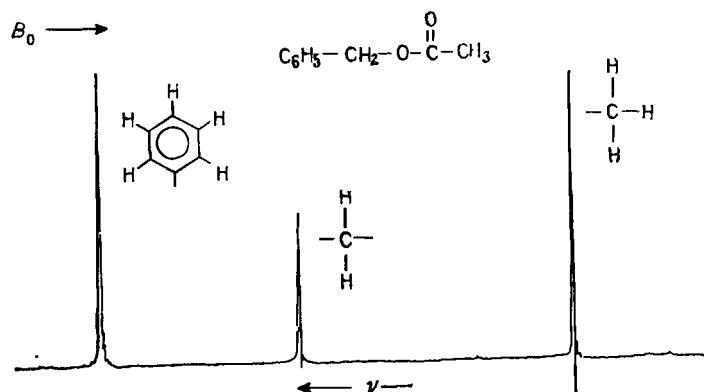
Рис. II. 1. Спектр протонного магнитного резонанса бензилацетата.
