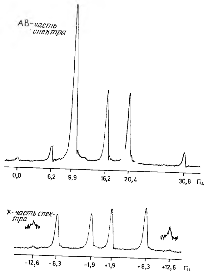
Рис. V.18. ABX-спектр алифатических протонов в L-аспарагине (при 100 МГц). X-часть расположена в более слабом поле.
