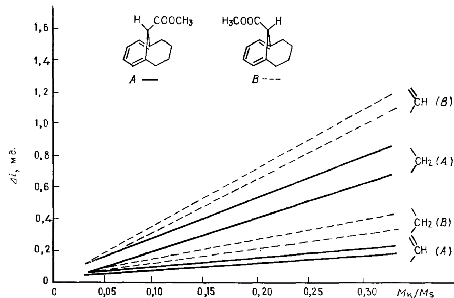
Рис. IX. 35. Псевдоконтактные сдвиги, индуцированные при добавлении Eu(FOD) 3 в спектре ЯМР 1 H экзо- и эндо-изомеров 11-карбоксиницикло[4,4,1]ундека-1,3,5-триена (Фишер [Fisher H., Diplomarbeit Universität Köln, 1978]).
