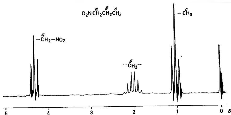
Рис. IV. 3. Спектр протонного магнитного резонанса 1-нитропропана.
