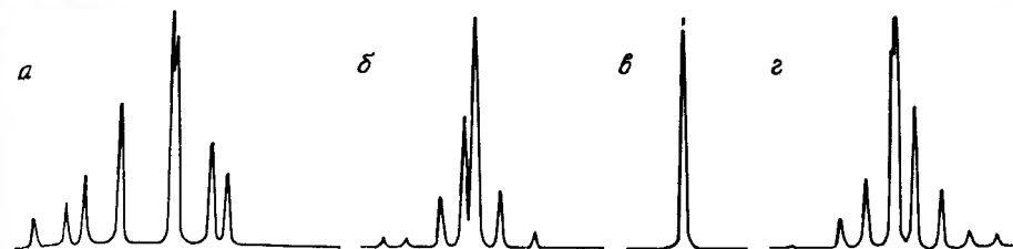
Рис. V. 8. Переход от системы АВ 2 к А 2 В-системе.
