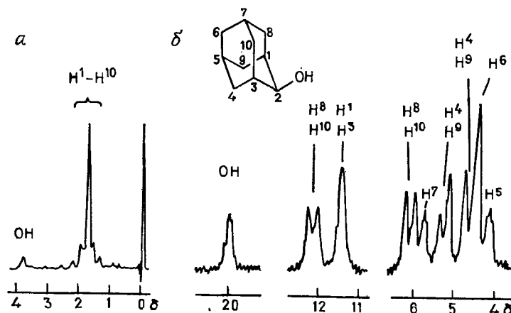
Рис. IX.34. Спектр ЯМР ^1\text{H} адмантанола-2 [16].
