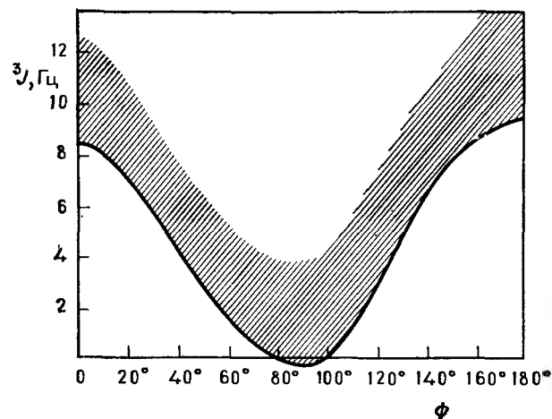
Рис. IV. 23. Кривая Карплуса — Конроя, описывающая зависимость вицинальной константы спин-спинового взаимодействия ^3J_{\text{HH}} от двугранного угла \phi . Сплошная линия — теоретическая кривая; заштрихованная площадь — область экспериментальных значений.
