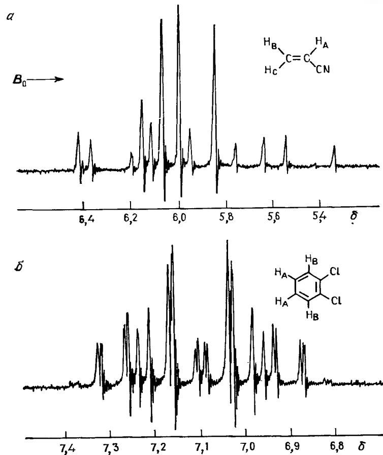
Рис. VI.3. Спектр ЯМР (60 МГц) акрилонитрила (а) и о -дихлорбензола (б).
