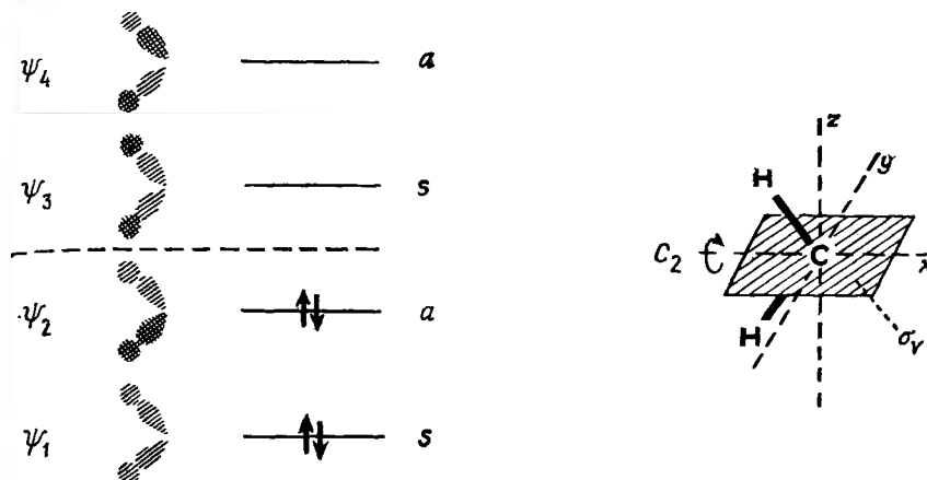
Рис. IV.22. Схема построения и диаграмма энергетических уровней молекулярных орбиталей группы CH_2 .
