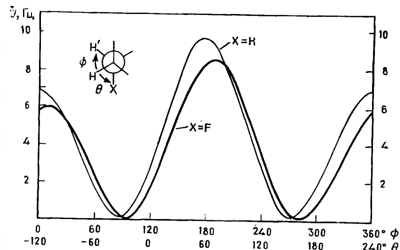
Рис. IV. 25. Влияние заместителя на вицинальную константу спин-спинового взаимодействия ^3J_{\text{HH}} в этане и этилфториде в зависимости от торсионного угла по результатам расчетов методом МО (Пахлер [12]).
