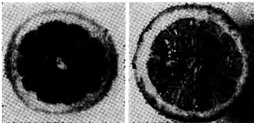
Рис. IX. 44. Слева. ^1\text{H} -ЯМР-изображение поперечного сечения лимона диаметром примерно 7 см. (С разрешения Эндрью и сотр. [22]).
