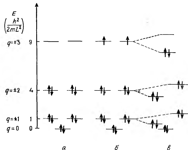
Рис. IV. 12. Диаграмма энергетических уровней для модели «электрон на окружности».
