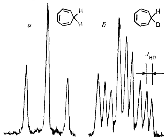
Рис. VI.12. Поглощение метиленовых протонов в спектрах ЯМР ^1\text{H} 1,3,5-циклогептатриена (а) и 7-дейтеро-1,3,5-циклогептатриена (б); |^2J_{\text{H,D}}| = 2,0 Гц, и по уравнению (VI.1) |^2J_{\text{H,H}}| = 13,0 Гц.
