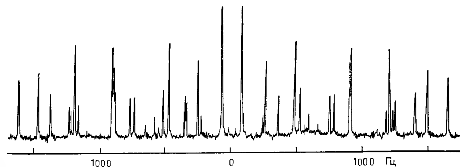
Рис. IX.39. Спектр ЯМР ^1\text{H} частично ориентированного бензола (Сауне [17]).
