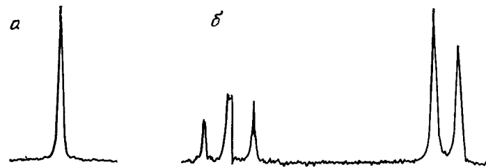
Рис. III.3. Концентрационная зависимость сигнала \text{CH}_2\text{OH} в бензиловом спирте в растворах ацетона.
