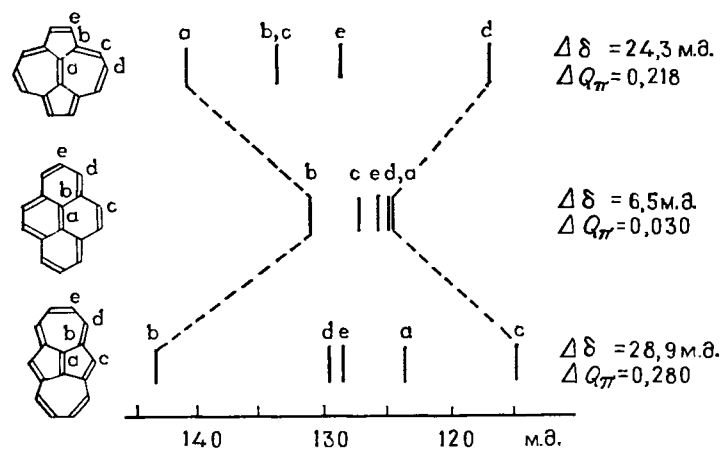
Рис. X.17. Химические сдвиги ^{13}\text{C} и разность зарядовой плотности в пирене и двух изомерных системах — дидекапентагепталене и дидекапентагепталене; значения \Delta Q_\pi рассчитаны методом ППДП/2 (Гюнтер, Шмиклер [12]).
