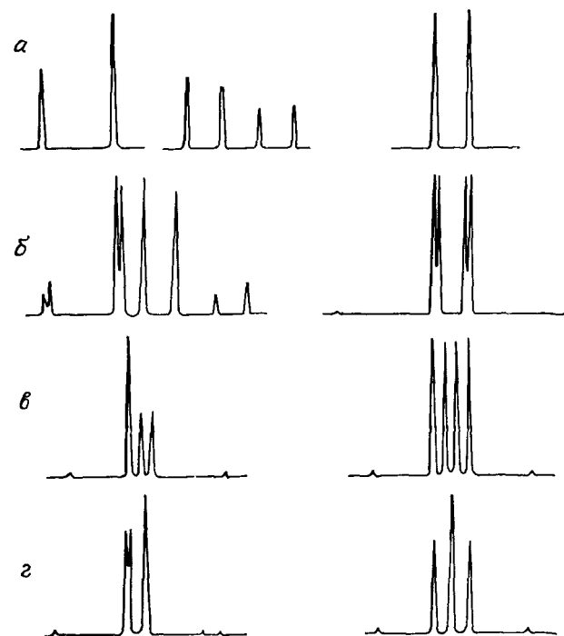
Рис. V. 17. Зависимость системы АВХ от параметра \nu_A - \nu_B . (Шлефер [3]).
