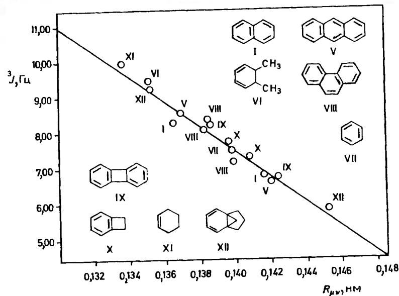
Рис. IV.24. Соотношение между вицинальной константой ^3J_{\text{HH}} и длиной связи R_{\mu\nu} в ненасыщенных шестичленных кольцах (Павличек, Гюнтер [11]). I — нафталин; V — антрацен; VI — цис -5,6-диметилциклогексадиен-1,3; VII — бензол; VIII — фенантрен; IX — бифенилен; X — бензоциклобутен; XI — циклогексен; XII — трицикло[4.3.1.0 4,6 ]декадиен-2,4.
