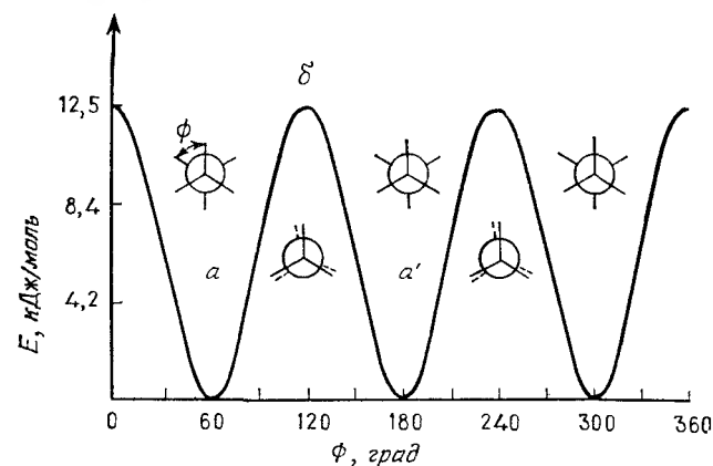
Рис. VIII.6. Профиль энергии для вращения вокруг углерод-углеродной связи в этане.
