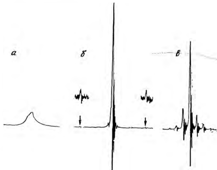
Рис. III. 5. Влияние вращения ампулы на форму резонансного сигнала. а — без вращения; б — с вращением; боковые полосы от вращения даны с усилением; в — с низкой скоростью вращения ( \sim 10 об./с).
