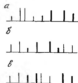
Рис. V. 15. Три типа АВ-частей спектров спиновых систем АВХ (см. текст).
