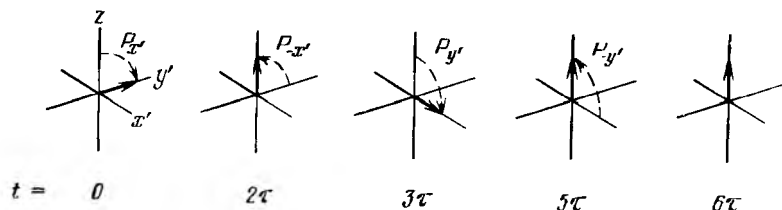
Рис. IX.41. Импульсная последовательность WALT16 для сужения линий в твердых телах при спиновом опрокидывании ( \text{Wo} и сотр. [19]).
