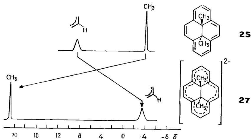
Рис. IV. 13. Сравнение спектров ЯМР аниуленов 25 и 27 с 14 и 16 \pi -электронами соответственно.
