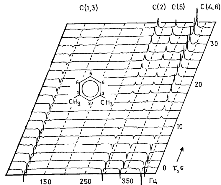
Рис. X. 9. Определение времени продольной релаксации T_1 ядер ^{13}\text{C} бензольного ядра m -ксилола (Бремзер и сотр. [6]). Для каждого спектра использовалась импульсная последовательность 180^\circ - \tau - 90^\circ , и \tau (в секундах) увеличивали с шагом 2 с.
