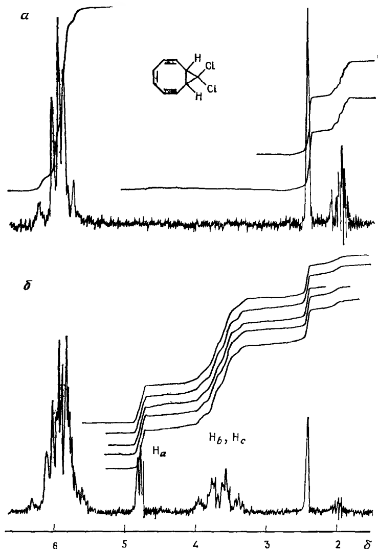
Рис. VIII.4. Спектры ЯМР ^1\text{H} для перегруппировки (138 \rightarrow 139) в ацетонитриле- d_3 .
